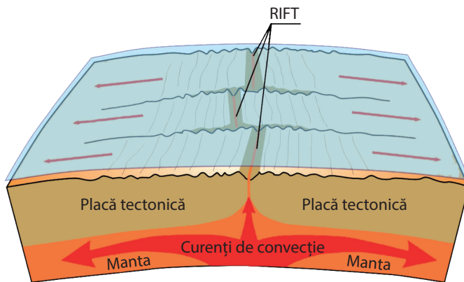
Plăcile tectonice se îndepărtează
